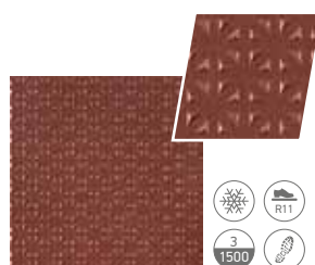
anti-slip tile Burgund F2 star противоскользящая плитка Бургунд F2 звезда 200×200×9 mm (3407)
