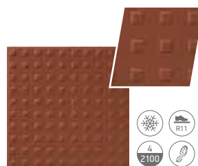
anti-slip tile Rot F1 square противоскользящая плитка Красная F1 квадрат 200×200×9 mm (0925)
