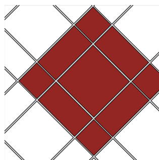
Layout 30×14,8 cm tile + 30×14,8 cm cut tile Укладывание плитка 30×14,8 см + резанная плитка 30×14,8 см
