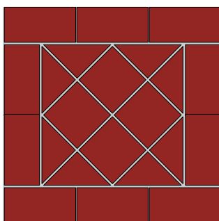
Layout 30×14,8 cm tile and 20×20 cm tile + 30×14,8 cm cut tile Укладывание плитка 30×14,8 см и 20×20 см + резанная плитка 30×14,8 см
