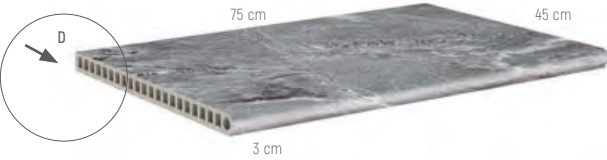
BORDE SKIMMER 45 x 75 x 3 cm - 17.7"x 29.5"x1.2" rectificado, rectified C-3
