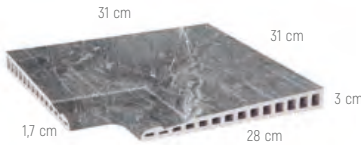
ÁNGULO DESBORDANTE 31 x 31 cm - 12.2"x12.2" rectificado, rectified C-3
