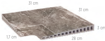
ÁNGULO DESBORDANTE 31 x 31 cm - 12.2"x12.2" rectificado, rectified C-3
